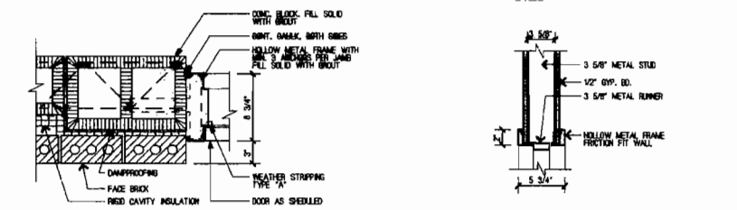
5 DOOR JAMB SCALE: 1 1/2"=1'-0" HMB/HMC
