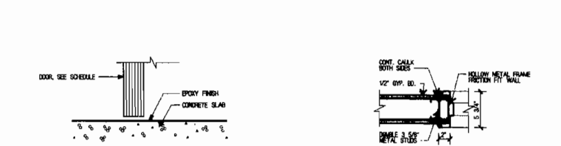
6 SILL SCALE: 3"=1'-0" CONC. - CONC.
